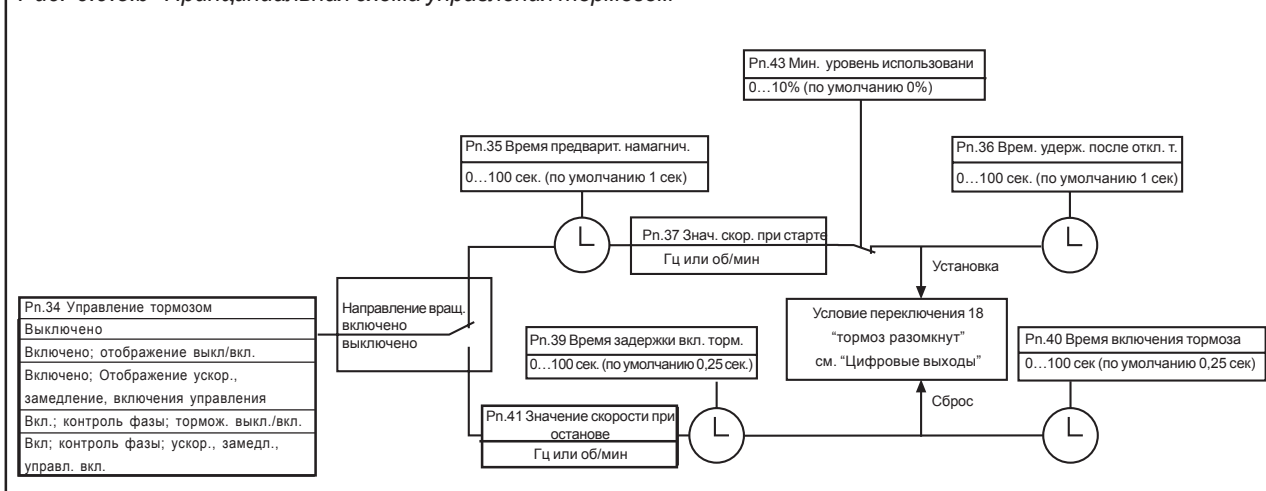
Рис. 6.9.5.b Принципиальная схема управления тормозом
