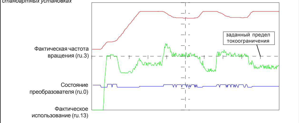
Рис. 6.7.2.в Действие функции опрокидывания (токоограничения) при стандартных установках
