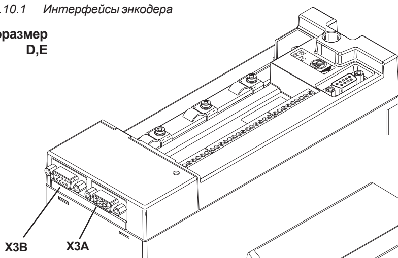
Рис. 6.10.1 Интерфейсы энкодера
