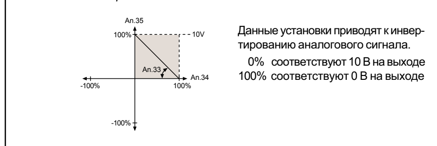
Рис. 6.2.14.б Инверсия аналогового выхода
