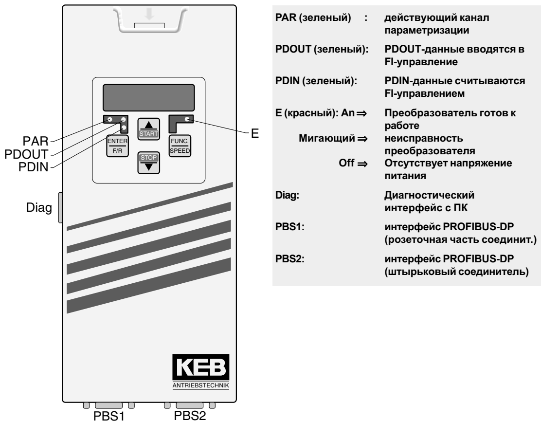
Рис. 11.1.5 Profibus-DP-Operator
