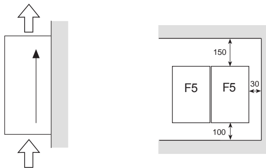
Направление охлаждения Минимальные расстояния
