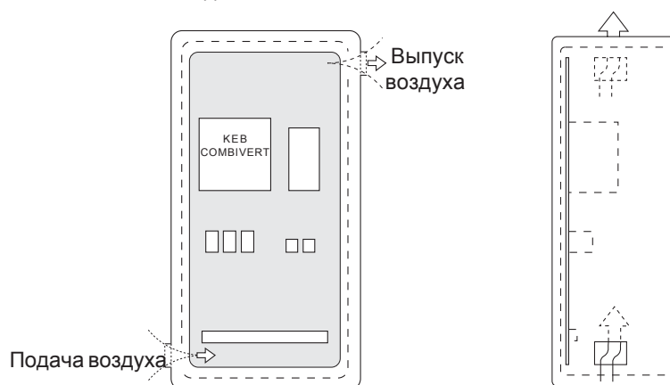
Направление охлаждения Минимальные расстояния
