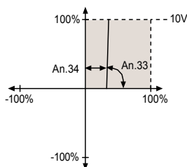
Рис. 6.2.14.с Аналоговый выход в качестве переключающего устройства
