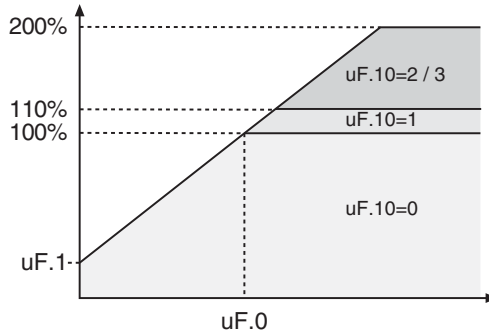
Рис. 6.5.2 Номинальная точка и Буст1.
