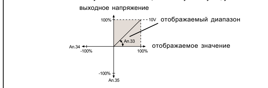
Рис. 6.2.14.а Заводская установка: смещение отсутствует, усиление 1
