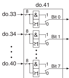
Рис. 6.3.20 Соединение выходов
