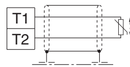
Датчик температуры (PTC) 1650 Ом...4 кОм сопротивление срабатывания 750 Ом...1650 Ом сопротивление сброса
