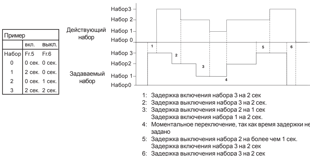
Рис. 6.8.9 Задержка включения/выключения
