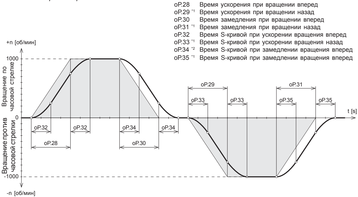
Рис. 6.4.6.a Время S-кривой
