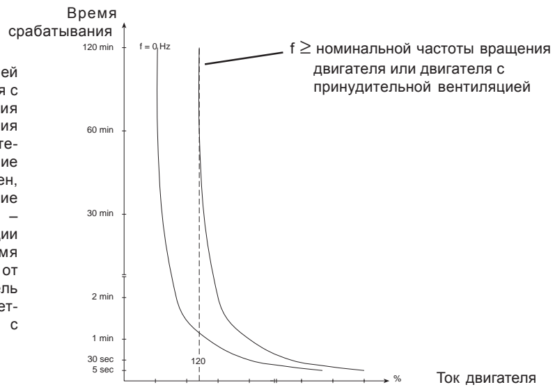
Рис. 6.7.8.b Время срабатывания функции защиты двигателя
